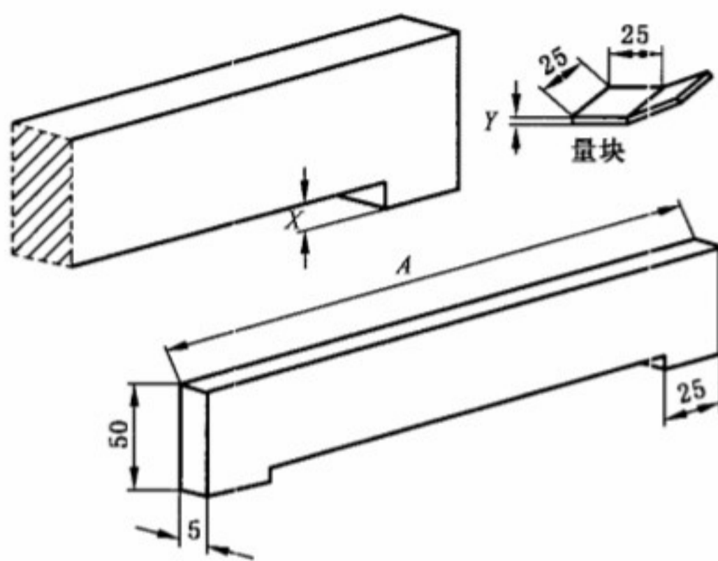
图 A.2 切口直尺和量规示例
